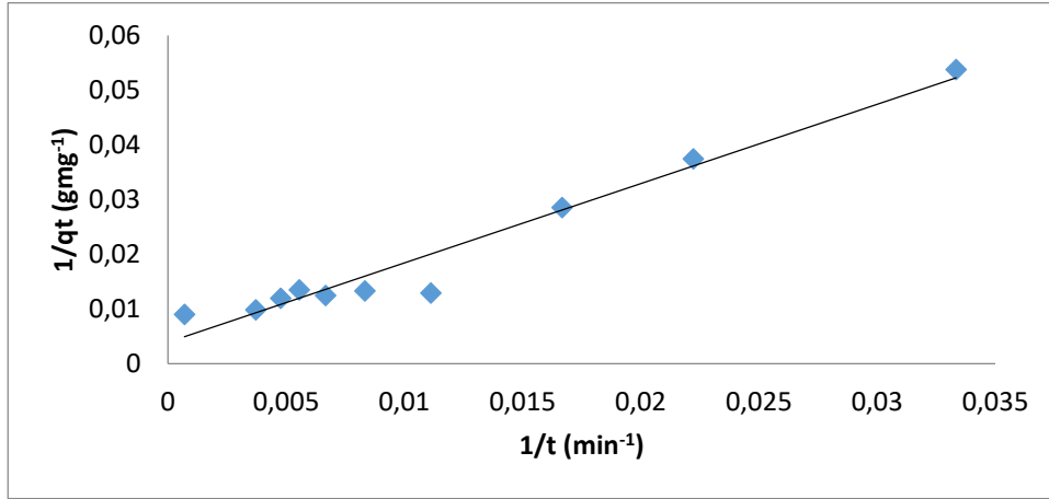
Şekil 5: Yalancı- ikinci dereceli kinetik model Tip 2 Grafiği
